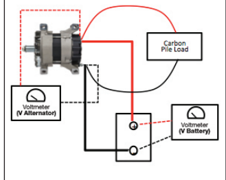
Figura 4B - Prueba del cable del alternador usando una pila de carbón
